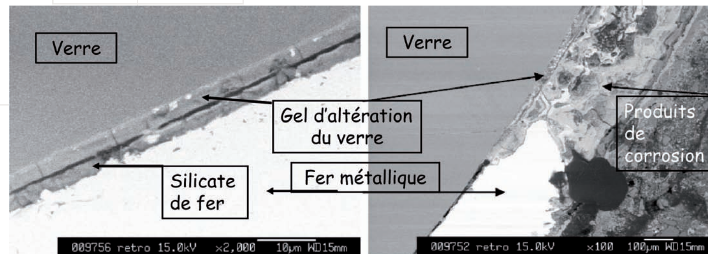
Figure 18 : altération du verre à l'interface verre/fer (à gauche) et au sein d'une fissure (à droite) dans l'expérience ArCorr 2006 (travaux CEA)
