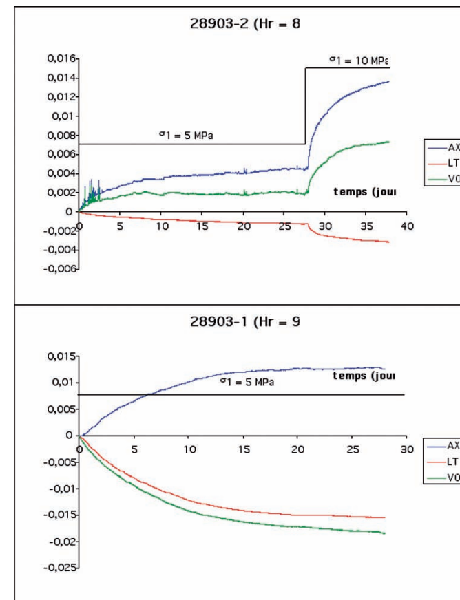
Figure 6 : évolution en fonction du temps des déformations obtenues en cours d'essais de fluage uni-axial à hygrométrie contrôlée
