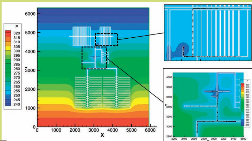
Exemple de résultats hydrauliques pour des écoulements orientés selon les galeries principales du stockage vers les puits de retour d'air
