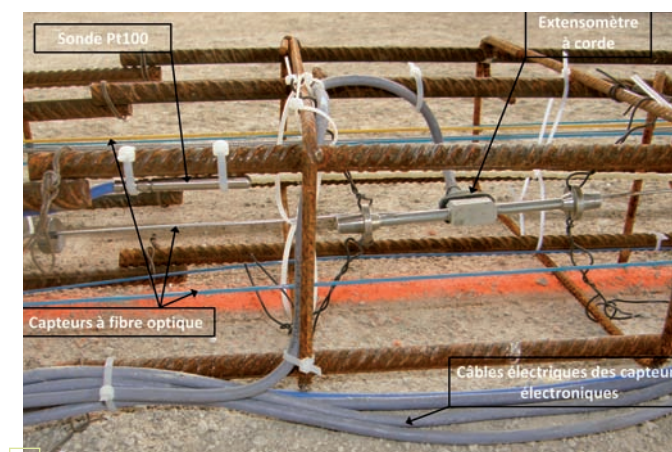
Figure 3 : ECV et capteurs à fibre optique avant coulage du béton dans un ouvrage pour mesures de température et de déformation
