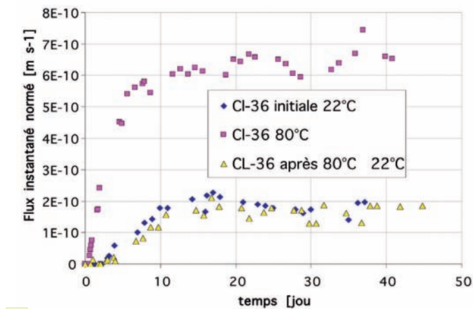
Figure 6 : comparaison des flux instantanés normés du Chlore-36 sur l'échantillon EST19496 (EST207, à 470m de profondeur) à 20°C, à 80°C et après le cycle thermique, à 20°C (d'après Savoye et al. , 2008)
