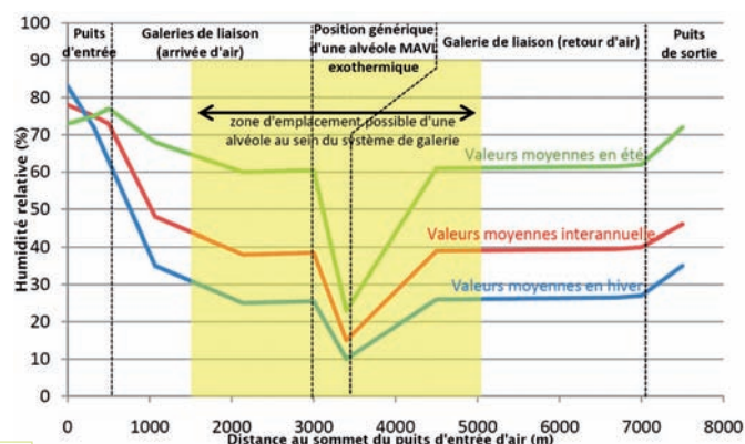
Figure 1 : évolution de l'humidité relative de l'air de ventilation du puits d'entrée d'air vers le puits de retour d'air via la zone de stockage MA-VL
