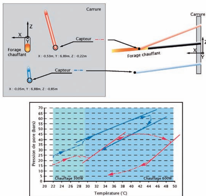
Figure 7 : configuration de l'expérimentation thermique TER et évolution de la pression de pore en deux points en fonction de la température
