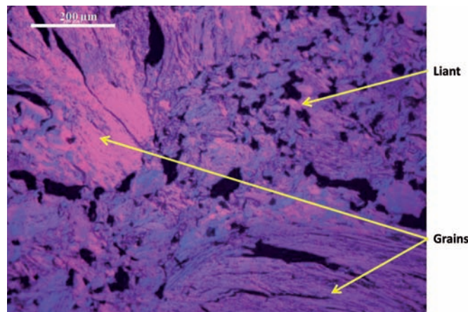
Figure 13 : observation au microscope optique polarisant du graphite vierge de Saint-Laurent A2. Le liant présente une porosité plus forte que les grains. (image ENS/CNRS)
