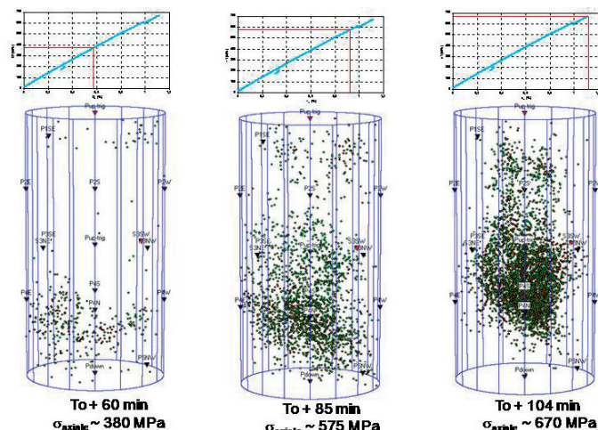
Figure 16 : synthèse des principales étapes d'endommagement d'un bloc de verre sain au cours d'un chargement déviatorique ( P_{conf} = 15 MPa) à travers l'enregistrement des émissions acoustiques. (Ougier et al. 2010)
