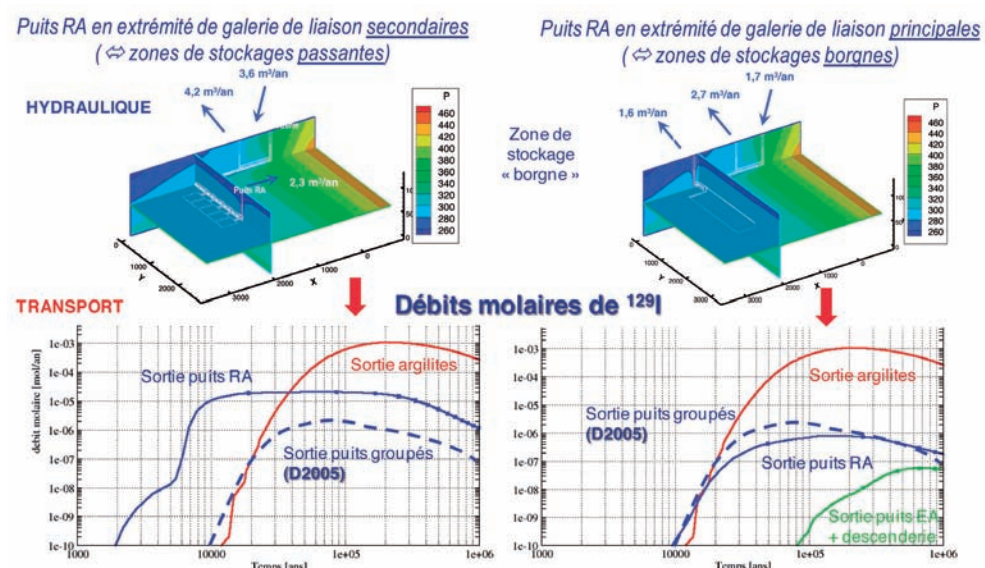
Figure 8 : déchets HA : évolution des débits molaires d'iode 129 en sortie des ouvrages et des argilites du Callovo-Oxfordien - Architecture « à puits de retour d'air dégroupés » étudiée pour le jalon 2009 : comparaison entre la situation avec zones de stockage passantes (à gauche) et celle avec zones de stockage borgnes (à droite)
