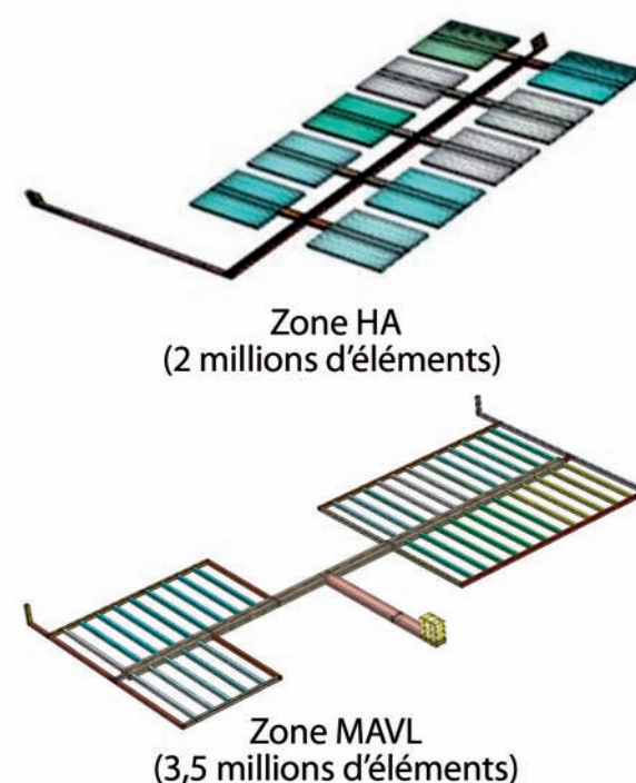
Figure 6 : exemples de maillages établis pour l'évaluation de performance des options de conception étudiées pour le jalon 2009. Traitement par zone séparée
