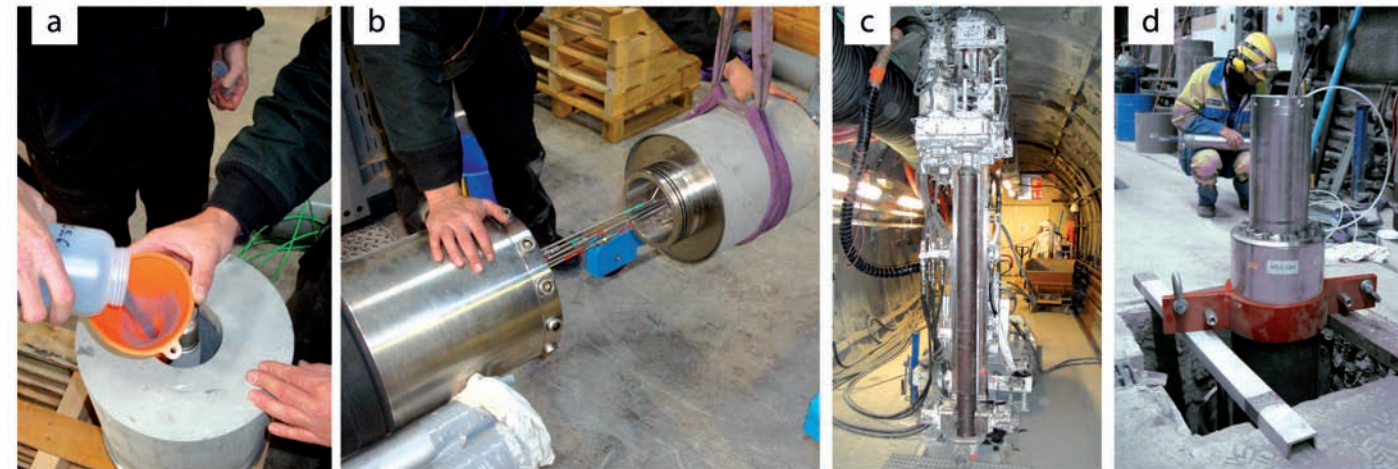
Figure 19 : installation de l'essai « MVE - long terme ». A- Remplissage de l'intervalle de la complétion avec le cylindre creux d'argilite et la poudre de verre B- Montage de la complétion (chambre de test + obturateur) C- Forage en Ø 350mm D- Mise en place de la complétion dans le forage
