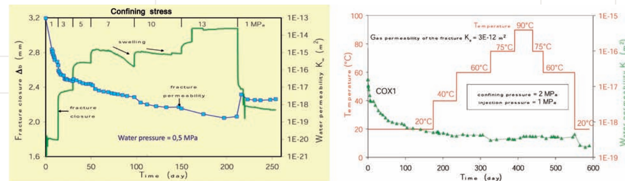
Figure 9 : diminution de la conductivité hydraulique d'une fracture, à gauche avec la resaturation et l'augmentation de contrainte, à droite malgré l'augmentation de la température (d'après GRS)
