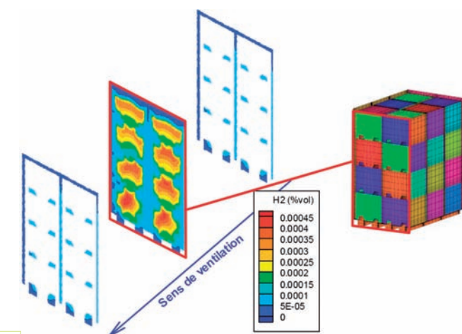
Figure 4 : valeur maximale de concentration en hydrogène dans une alvéole MA-VL pleine avec une ventilation de 3 m³/s
