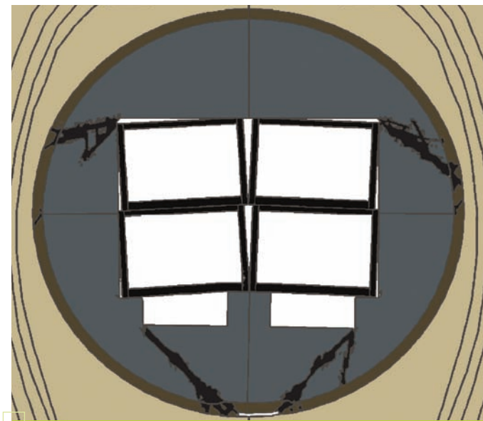
Figure 5 : simulation de l'évolution mécanique d'une alvéole MA-VL à 100 000 ans
