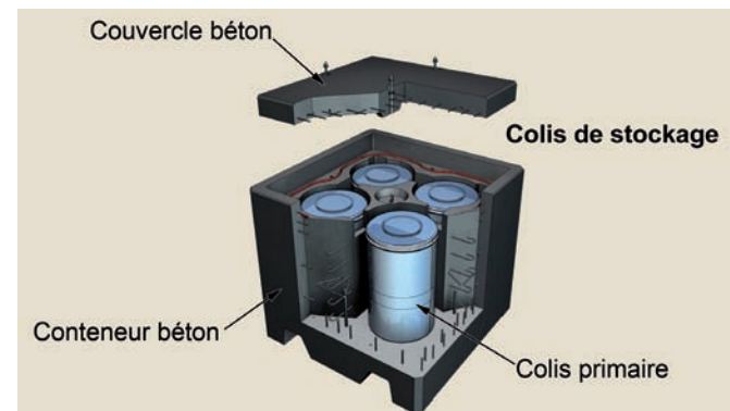
Figure 10 : exemple de surconteneur béton prévu pour le stockage contenant quatre colis primaires de déchets MA-VL
