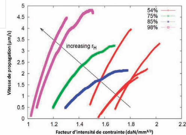
Figure 4 : exemple de résultats d'essais de propagation de fissures par relaxation de contrainte lors d'essais de double torsion
