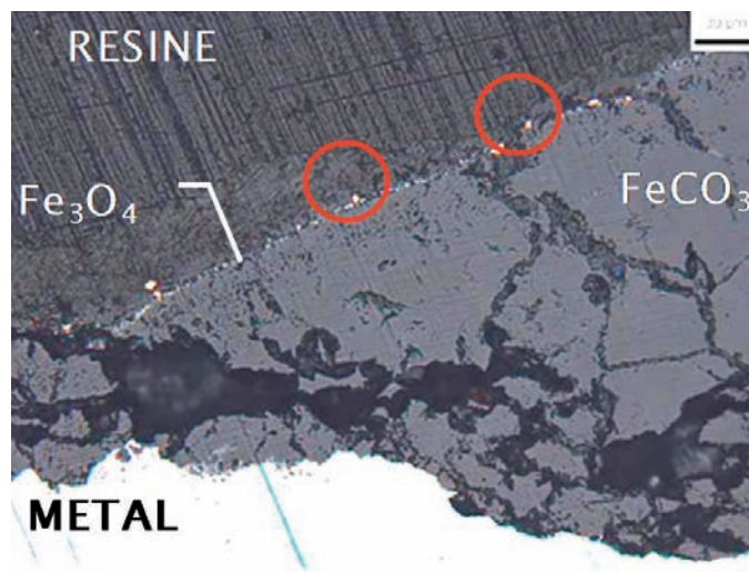
Figure 20 : réduction du cuivre sur les produits de corrosion pour identifier les zones de réaction cathodique (cercles rouges) - Travaux du CEA/LAPA
