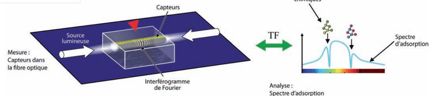
Figure 2 : capteur à fibre optique exploitant l'absorption du spectre lumineux pour identifier et quantifier la présence de certaines molécules
