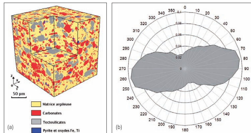
Figure 3 (a) distribution spatiale des minéraux déterminé par microtomographie synchrotron (coté cube ~150µm) (b) rosace d'orientation des grains de carbonate relative au plan de sédimentation (90°)
