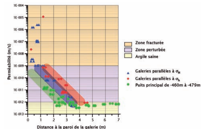
Figure 5 : compilation de mesures de perméabilité autour des ouvrages du Laboratoire souterrain. Les essais ont été réalisés au gaz sur le premier mètre du fait de la désaturation de l'argilite
