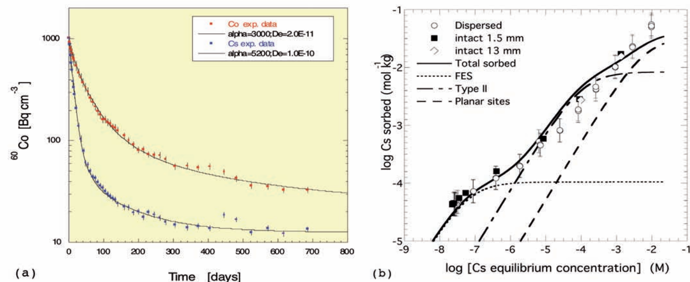
Figure 4 : (a) concentration en Co et Cs en solution lors de l'équilibration avec une pastille de l'argile à Opalinus. - (b) Isothermes de sorption pour Cs (argile à Opalinus) en forme broyée, pour 2 systèmes à roche intacte. Le trait plein correspond à l'isotherme calculé avec un modèle thermodynamique (Jakob et al. , 2009)
