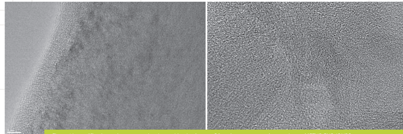
Figure 14 : modifications microstructurales du graphite du réacteur G2 après passage en réacteur. Image METHR ENS/CNRS. La plupart des zones restent bien organisées (à gauche) même si quelques rares zones sont désorganisées (à droite)
