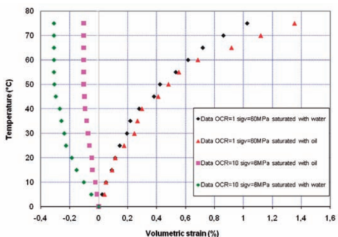
Figure 8 : déformations volumiques résultant de chargements thermiques sur échantillons d'argilite massive
