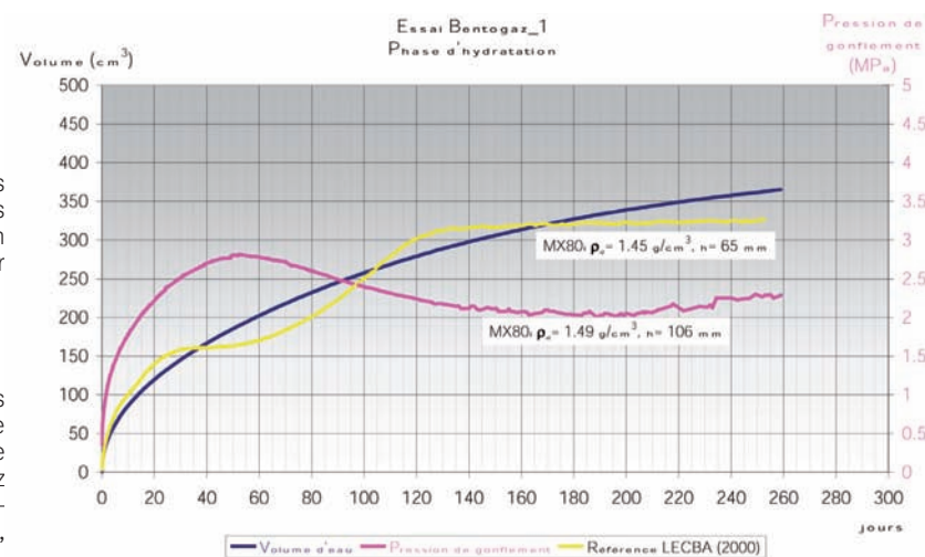
Figure 10 : évolutions de la pression de gonflement au cours de la phase de resaturation d'un mélange pellets/poudre
