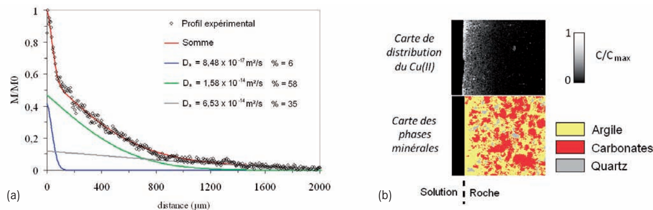
Figure 5 : (a) profil de Cu(II) dans l'argilite du Callovo-Oxfordien, en partant de la surface en contact avec la solution ( x = 0 ), avec courbes d'ajustement de D_a ( \sim D_e/K_d ). - (b) Comparaison de la carte minérale (en bas) et de la distribution du Cu (en haut) ; la carte minérale montre la déstructuration importante du bord de l'échantillon en contact avec la solution (Robinet, 2008).
