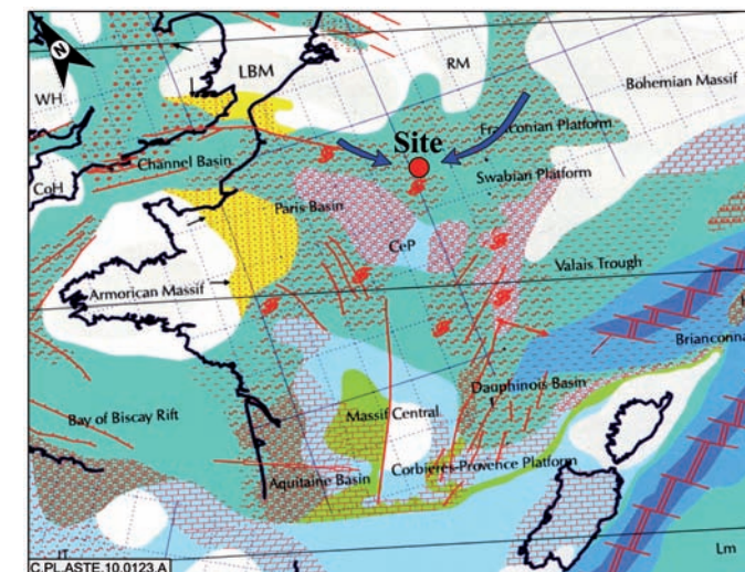
Figure 4 : position du site par rapport aux massifs émergés (en blanc) au Callovien - Extrait de Thierry J. et Borrier E - map 9 - in Atlas Péri-Téthys - 2000 LBM : massif de Londres - Brabant
