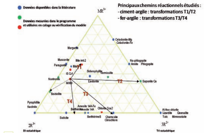
Figure 1 : diagramme ternaire de composition des minéraux argileux. Indication des chemins réactionnels correspondant à des processus attendus en stockage
