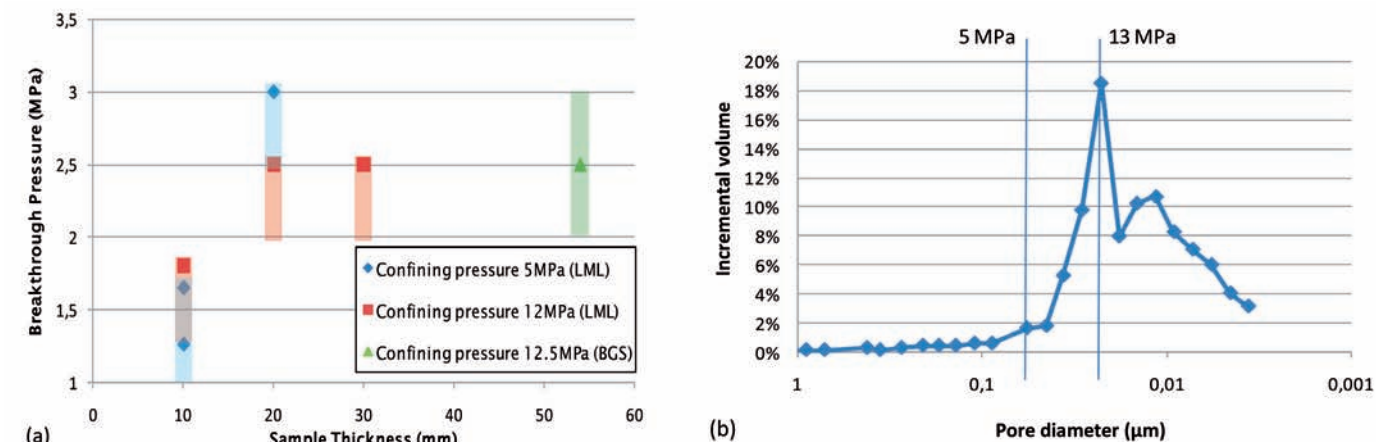
Figure 8 : (a) mesures de pression d'entrée de gaz, (b) porosimétrie au mercure (indication des pressions d'entrée de gaz équivalentes pour un système eau/gaz)
