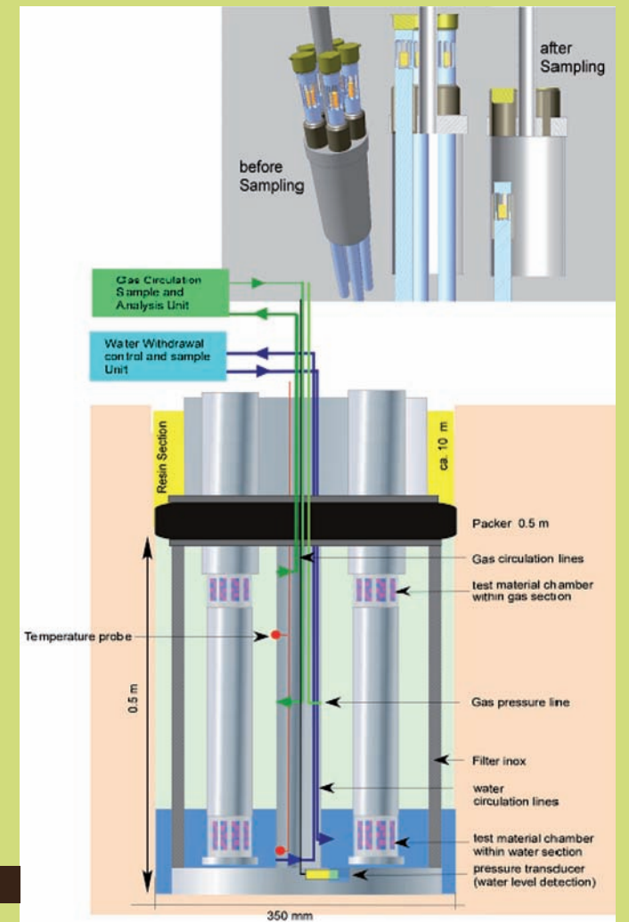
Schéma du dispositif expérimental pour l'essai MCO
