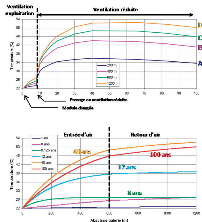
Figure 2 : évolution de la température de l'air de ventilation dans l'espace et dans le temps dans un module HA
