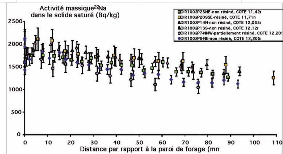
Figure 2 : profils de diffusion du 22 Na dans l'argilite à 490 m de profondeur
