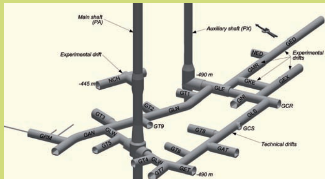
Vue du réseau de galeries en janvier 2010
