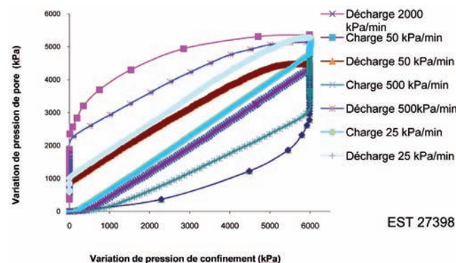
Figure 3 : réponses en pression de pore lors du premier essai en compression non drainée
