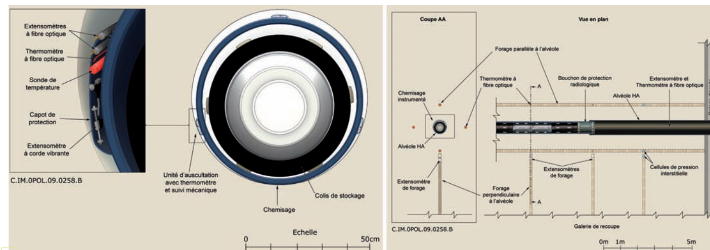
Figure 1 : exemple de dispositions prévues pour l'observation-surveillance d'alvéoles HA
