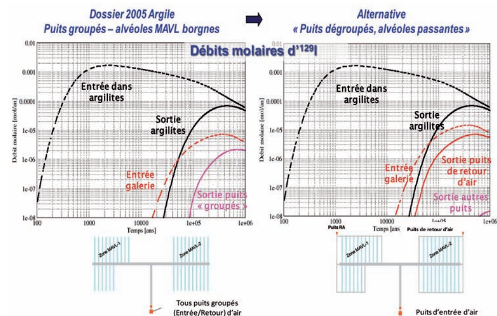
Figure 9 : déchets MA-VL : évolution des débits molaires d'iode 129 en sortie des ouvrages et du Callovo-Oxfordien (argilites) - comparaison entre l'architecture « à puits groupés et alvéoles borgnes » du Dossier 2005 Argile (à gauche) et l'architecture « à puits de retour d'air dégroupés et distants » avec alvéoles passantes étudiée pour le jalon 2009 (à droite)
