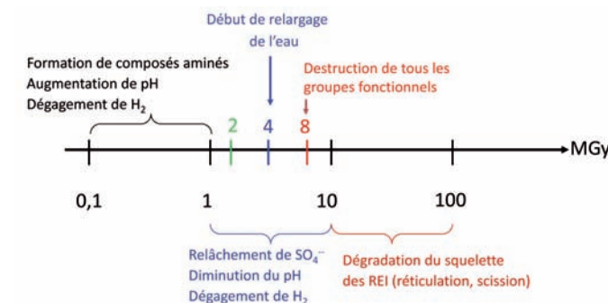
Figure 15 : comportement sous irradiation des REI utilisées dans le démantèlement des réacteurs UNGG
