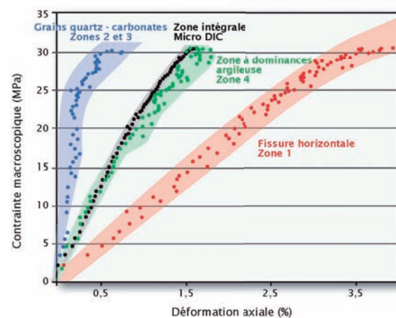
Figure 2 : mesure de la déformation locale dans un échantillon d'argilite à partir d'une image micro-DIC (d'après LMS)
