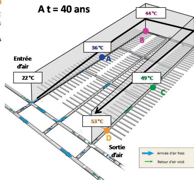
Figure 2 : évolution de la température de l'air de ventilation dans l'espace et dans le temps dans un module HA
