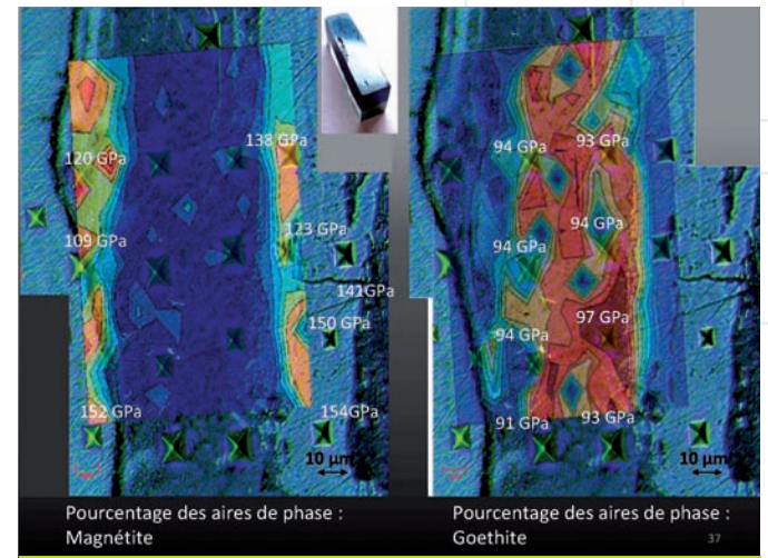
Figure 12 : superposition d'analyses par micro-indentation et analyses Raman d'une couche de produits de corrosion. Modules d'Young en GPa vs domaines de concentration en magnétite (à gauche) ou en goéthite (à droite) ; la proportion est d'autant plus élevée que la teinte est rouge
