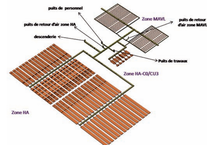
Figure 7 : exemple de maillage établi pour l'évaluation de performance des options de conception étudiées pour le jalon 2009. Traitement du stockage en grand
