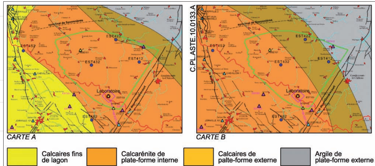
Figure 5 : cartes paléogéographiques du Bathonien (carte a, à gauche) et de la transition Bathonien Callovien (carte b, à droite)
