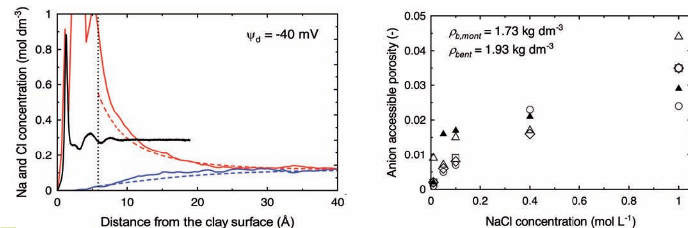
Figure 10 : à gauche, distributions de Cl - (bleu) et Na + (rouge) calculées par DM (trait plein) et avec un modèle TCE (traits en pointillé) - le trait noir correspond aux molécules H 2 O. À droite, comparaison des prédictions des effets de l'exclusion anionique par le modèle TCE (triangles solides) avec des mesures expérimentales pour une montmorillonite compactée, en fonction de la force ionique et la densité de l'argile (Tournassat et al. 2009)
